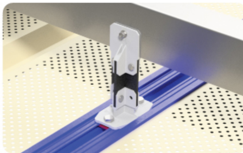
열교 차단 포스트
