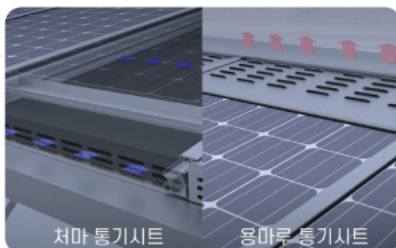
모듈 배면 통풍로
