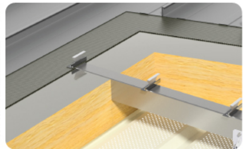
방수 패킹재, 슬라이딩 클립
