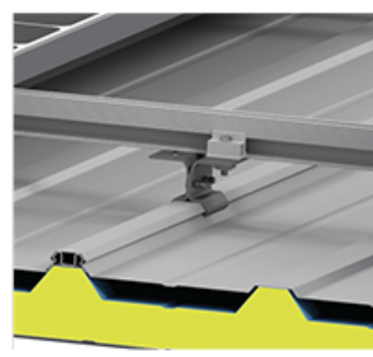
[ 모듈 부하 하중 분산 ] 태양광 구조연결부
